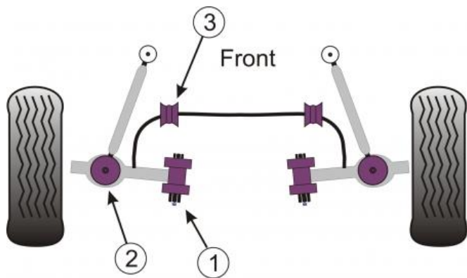
Porsche Cayman 987
